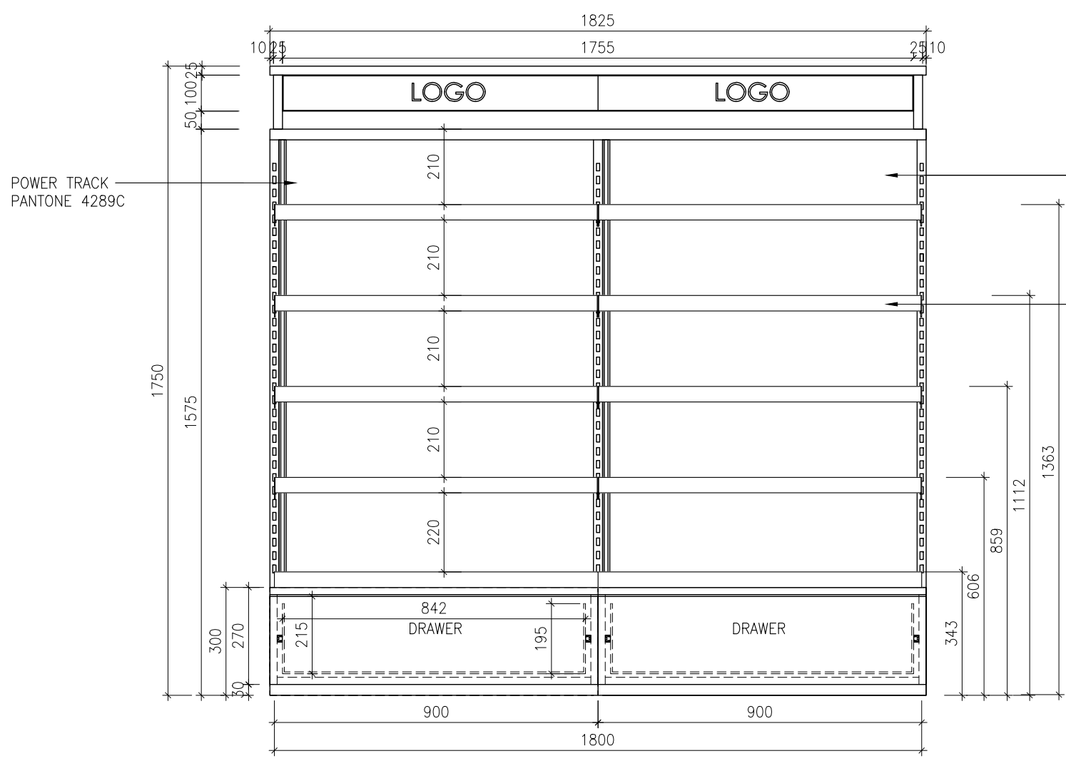
2 ELEVATION 1 SCALE 1:15
