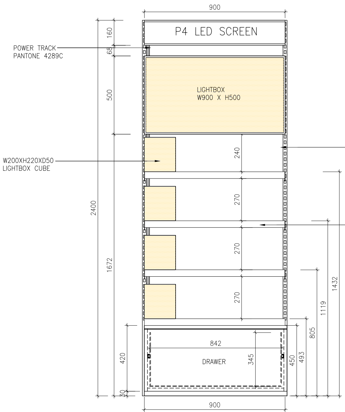
2 ELEVATION 1 SCALE 1:15
