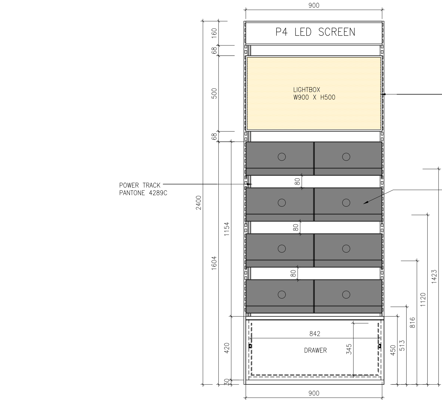
2 ELEVATION 1 SCALE 1:15
